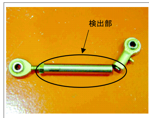
7-2 破損した初期型センサ（約10時間使用后）
