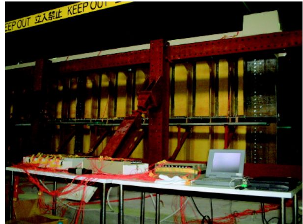
図2 歪測定装置
