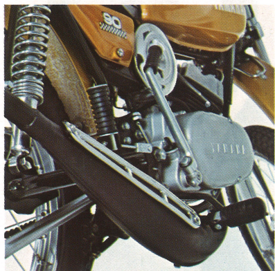
材質、形状とも一新して操作しやすくなったキック。ワイルドなダウンマフラー。
