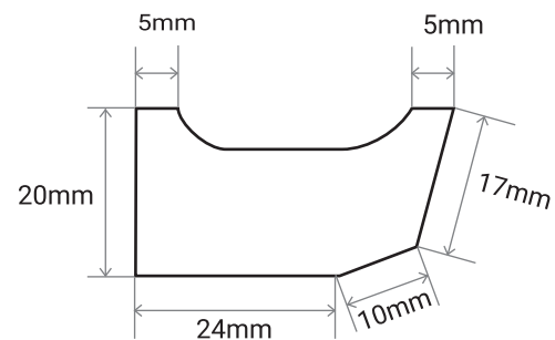
D 厚さ 25mm
