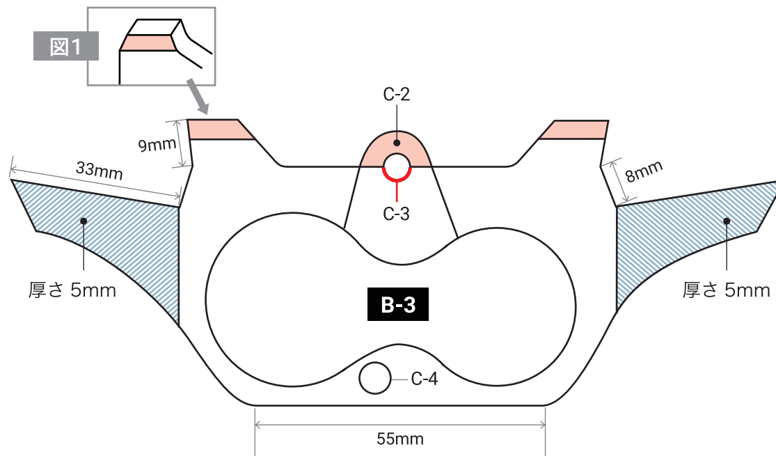
C キャリパーボディー 厚さ 9mm
