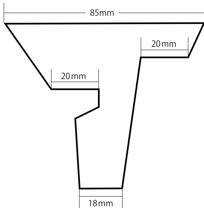
型紙 C 高さ 15mm
