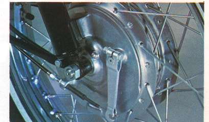
雨やホコリにも強い防塵防水ブレーキ
