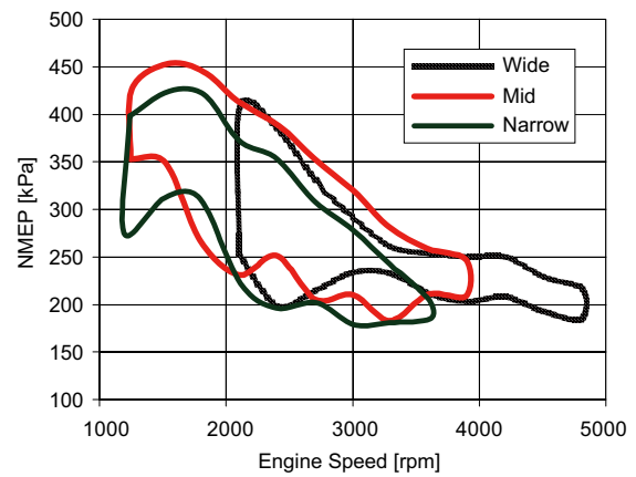
図9 運転領域
