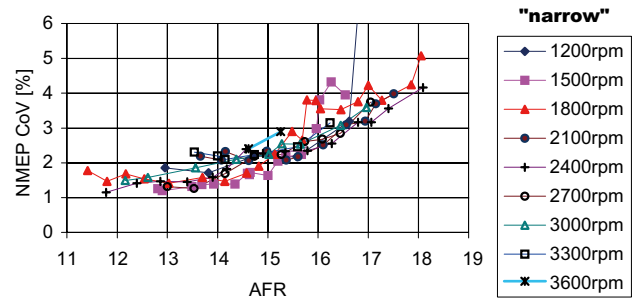
図12 燃焼変動率
