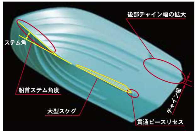
図 5 船型概念図
