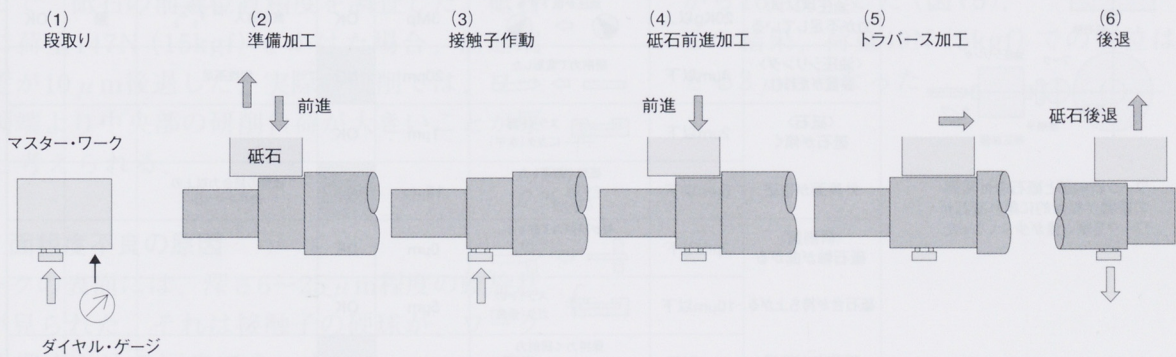
図10 研削手順
