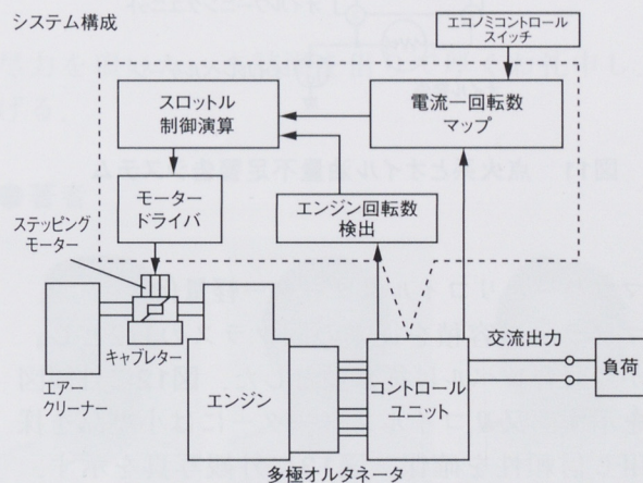
図9 電子ガバナークシステム図
