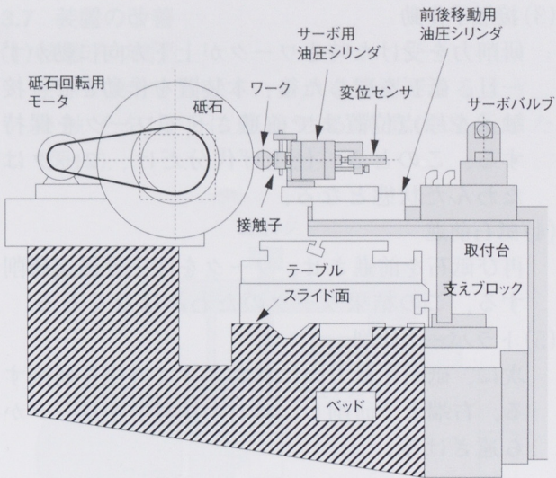
図9 装置の概観
