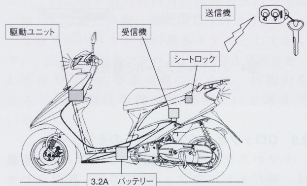
図3 リモコンシステム
