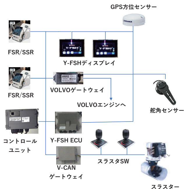
図4 Y-FSH システム図
