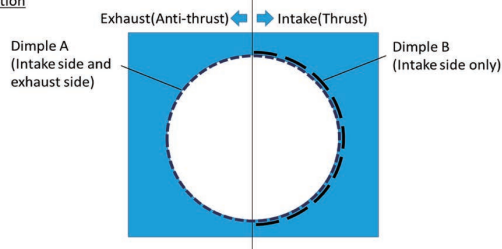
図4 ディンプル付与範囲の模式図
