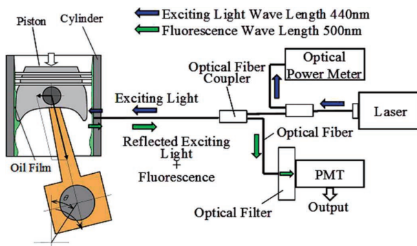
図2 レーザー誘起蛍光法 (LIF 法) による油膜測定の概略図
