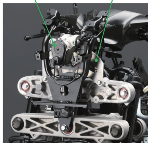
図5 電動キャリパとディスクプレート
