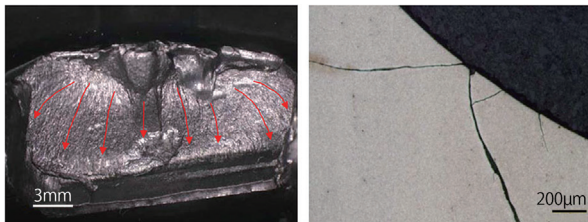
隅R形状部を起点とする放射状模 および疲労破壊の特徴である貝殻 模様が見られる 上側に進行するクラックと下側 に進行する複数のクラックが交 わっている
