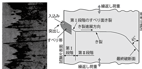
図6 高力アルミニウム合金平滑材の疲労で観察される種々の破壊形態 [1]
