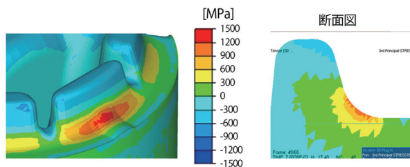
図5 破損部位の最大主応力分布
