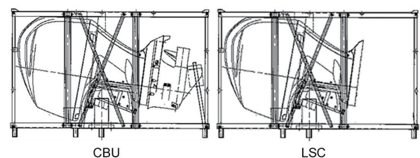
図8 CBUとLSCの梱包仕様（F350A）
