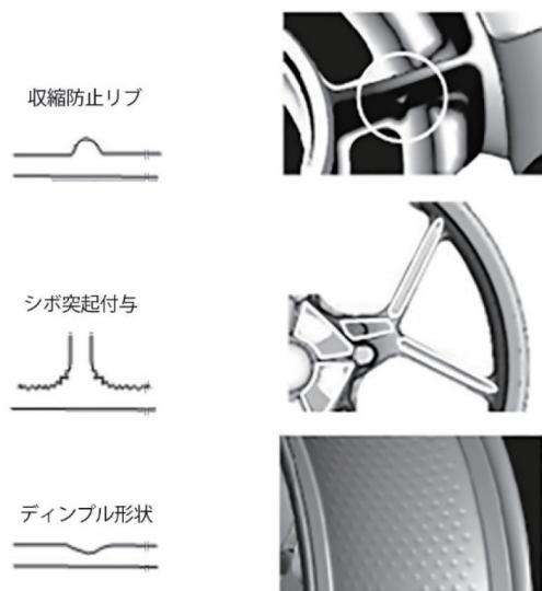
図13 ホイール設計時に採用した製品形状
