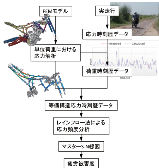
図8 疲労解析プロセス
