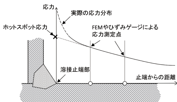
図2 ホットスポット応力の定義
