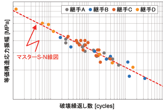
図7 等価構造応力と破壊繰返し数の関係
