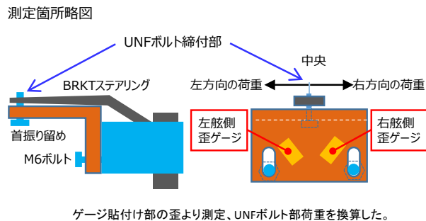
図5 首振り留めの荷重測定方法
