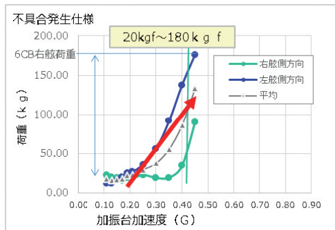
図6【不具合発生仕様】加速度と荷重変化の関係
