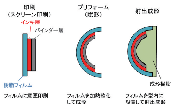
図2 インサートグラフィック工法
