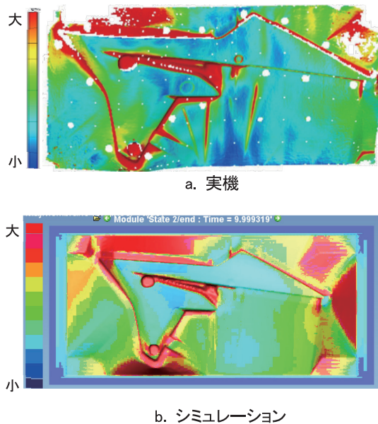
図9 フィルムひずみ比較
