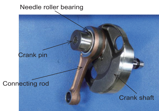
図1 分割型クランクシャフト
