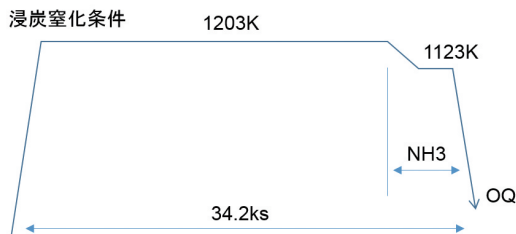
図4 Harrisの実験式
