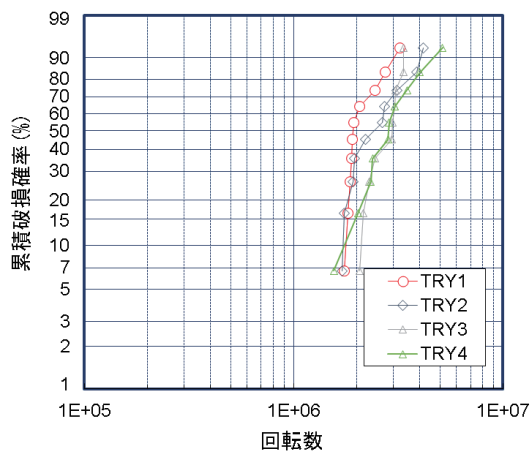
図7 浸炭窒化実験結果
