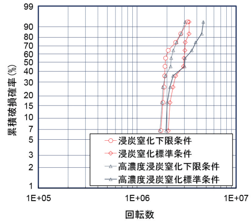
図9 ワイブル分布(工法比較)
