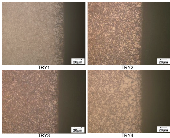
図7 浸炭窒化実験結果
