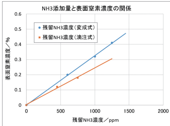
図11 添加NH3と窒素濃度の関係
