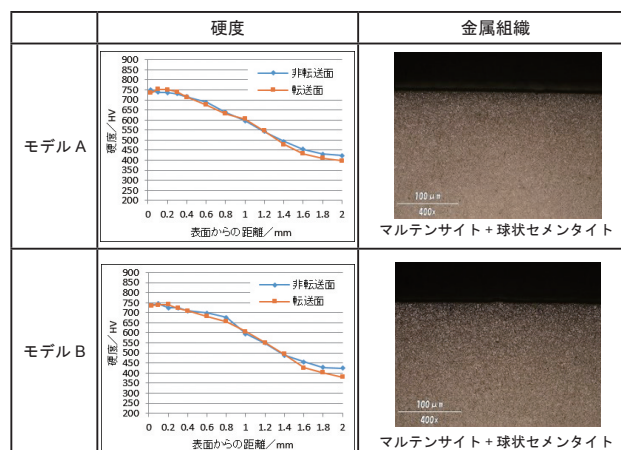
図3 硬度、金属組織測定結果
