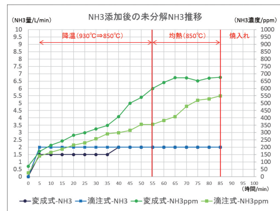
図10 アンモニア濃度の推移
