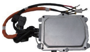
図8 パワーユニット、モーターコントロールユニット
