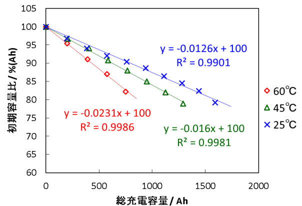
図4 サイクル劣化評価結果例と劣化係数の算出
