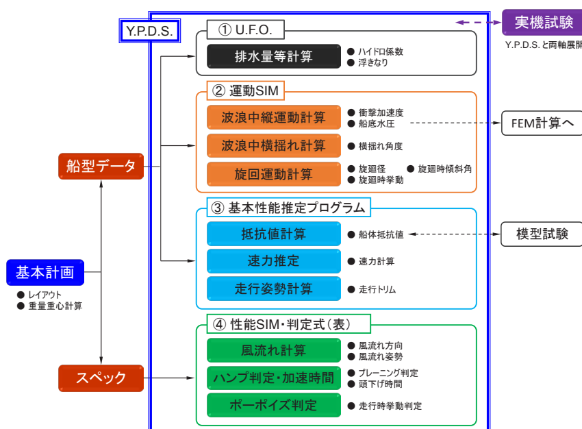
図5 Y.P.D.S. 概要図
