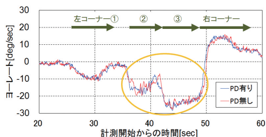
図6 実走行中のヨーレート
