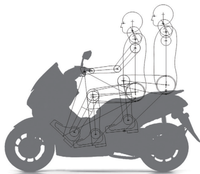
図7 ライディングポジション
