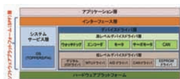
図3 ECUプラットフォームの構造
