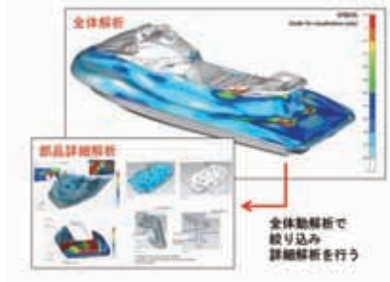
図 8 動解析例
