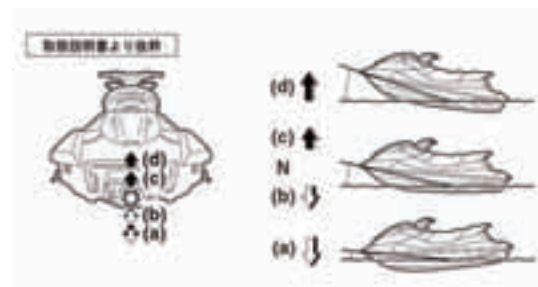
図 14 トリム機構
