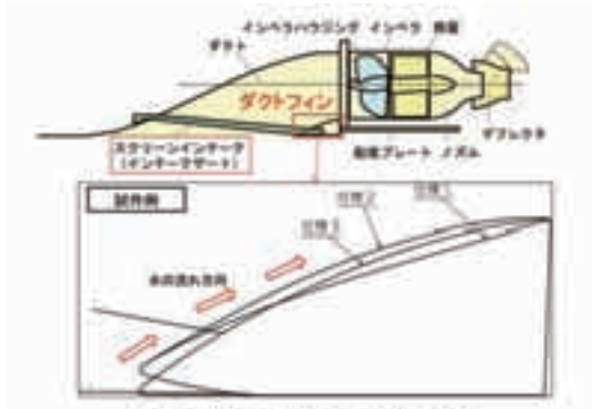
図 10 スクリーンインテークとダクトフィン形状
