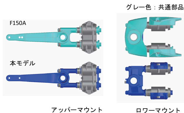
図6 マウント形状比較
