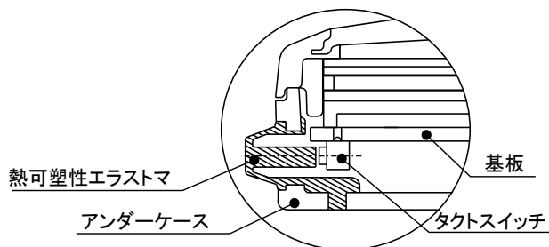
図7 横押しスイッチの構成
