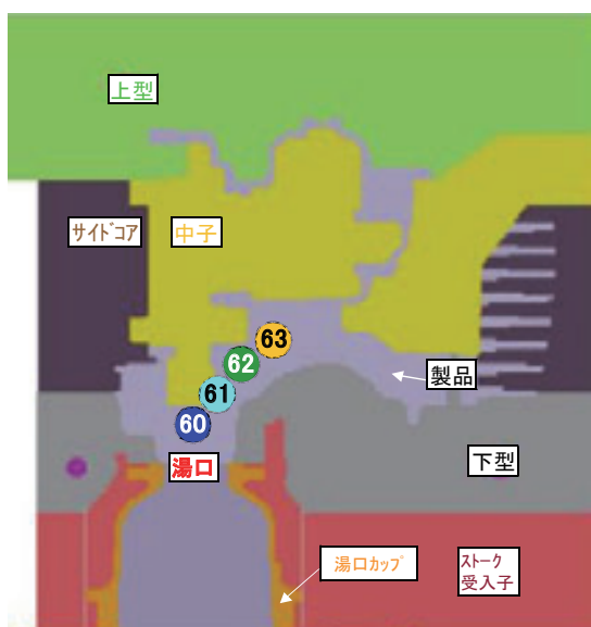
図 16 製品内センサー位置
