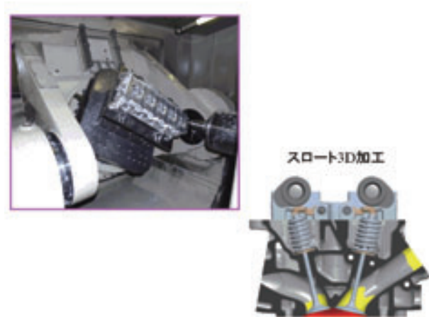
図7 3D加工
