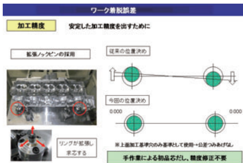
図6 ワーク脱着誤差
