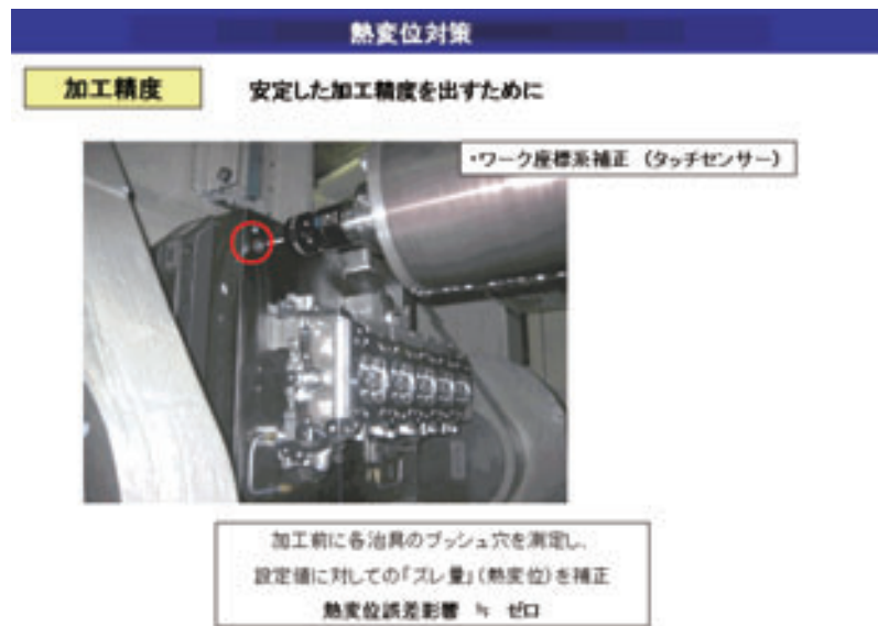
図5 熱変位対策
