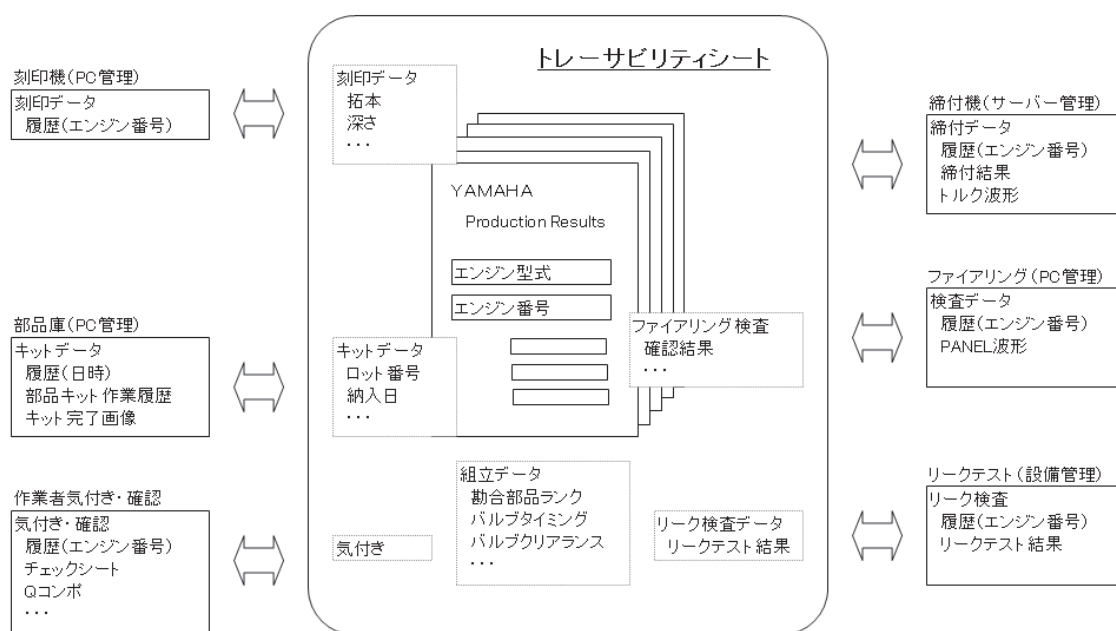
図 18 組立のトレーサビリティ体系イメージ図
