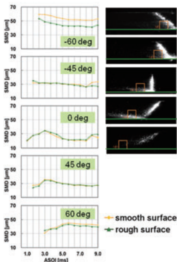
Fig. 21 Temporal variation of SMD value in area (d) with low ambient flow
