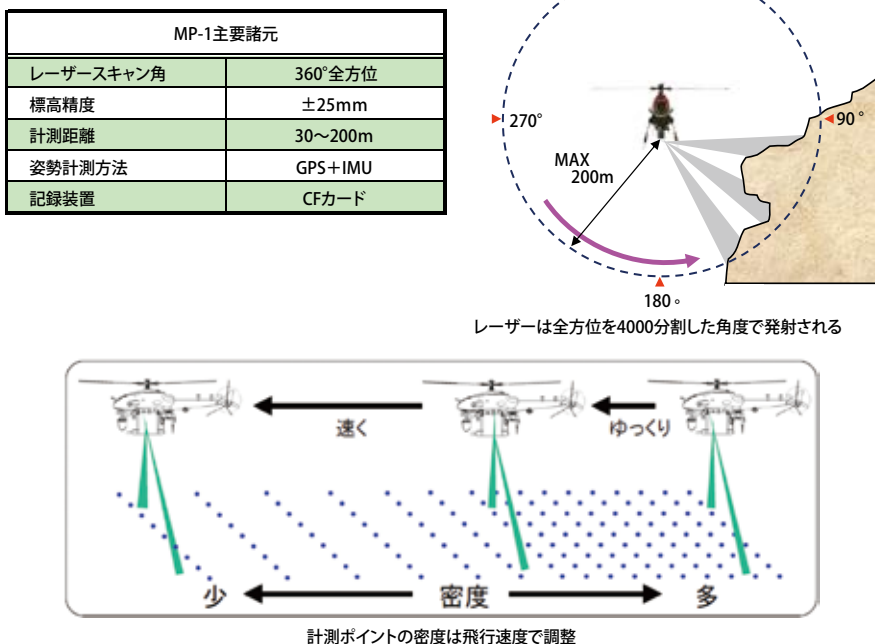
図6 MP-1 主要諸元
