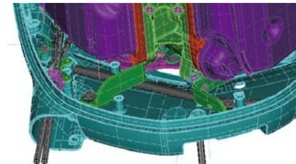
図4-6 ボトムカウルの吊下げ構造
