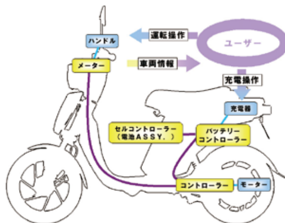
図4 システム図
