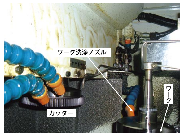
図 20 ワーク洗浄システム
