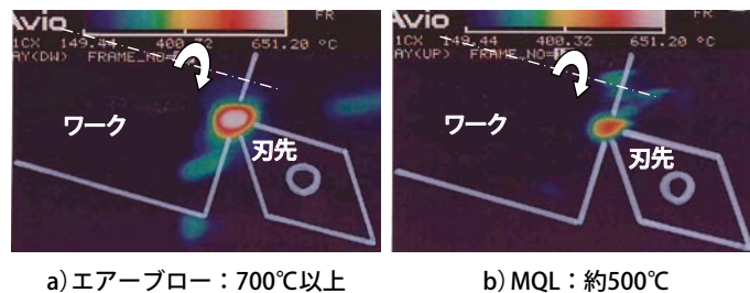
図8 冷却の制御：刃先付近の切屑の温度
