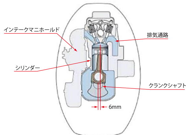
図3 オフセットクランクシャフト
