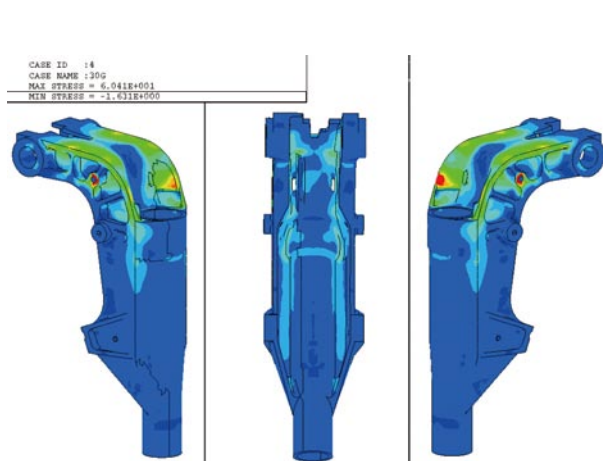
図 12 ブラケット強度解析例
