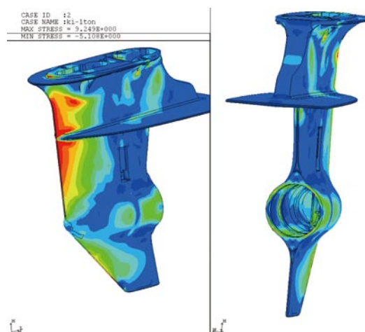
図 13 ロワーケース強度解析例
