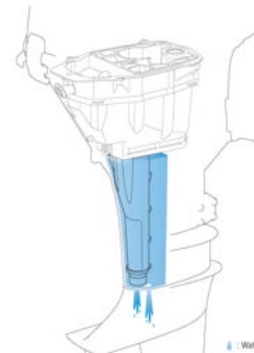
図11 アッパーケース水壁構造
