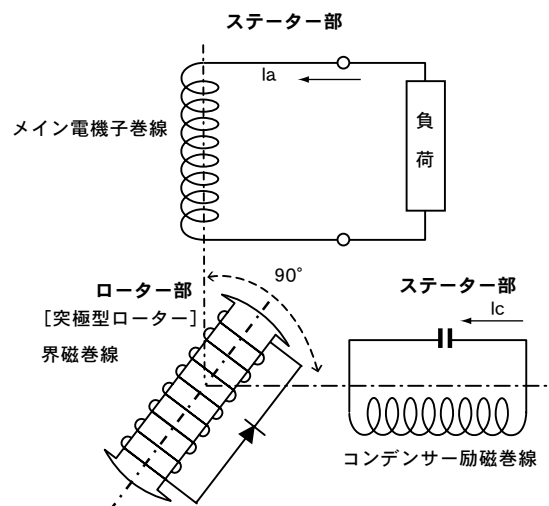
図4 コンデンサー補償式回路図(ET500)
