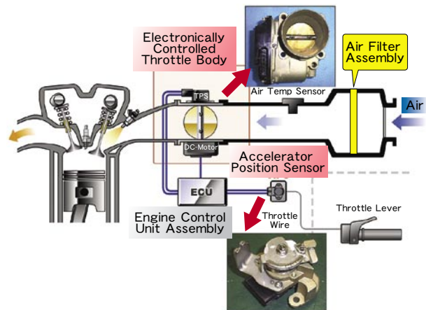
図11 システム図
