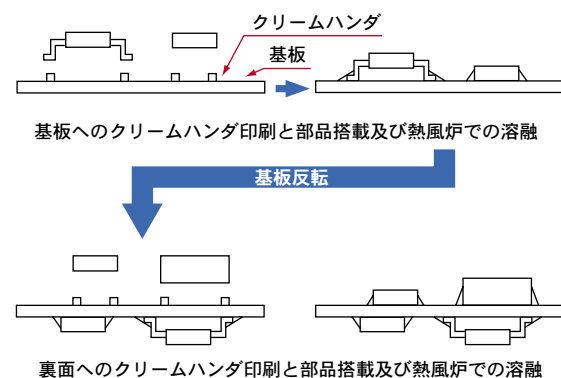
図3 リフローソルダリング工程
