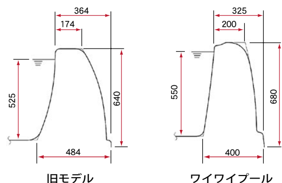
図9 側壁の断面図
