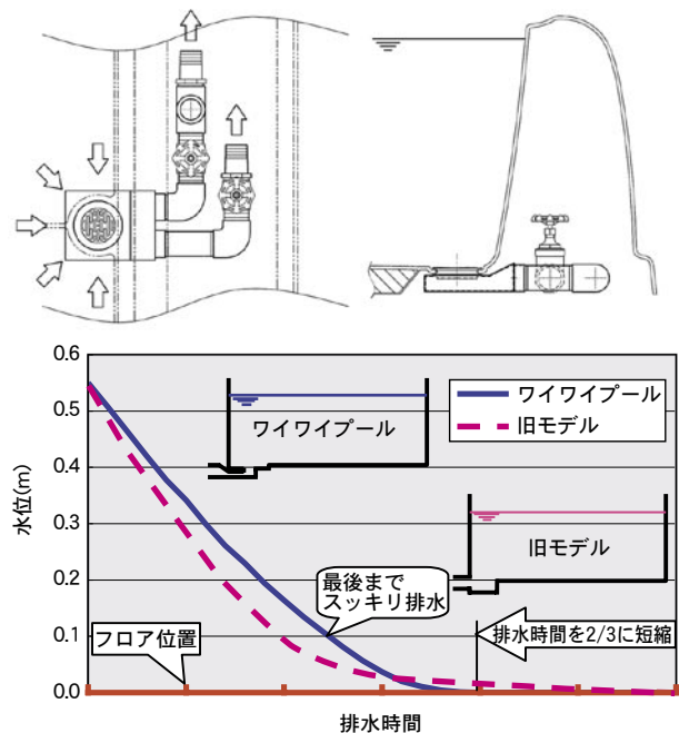
図5 排水構造と排水時間の比較
