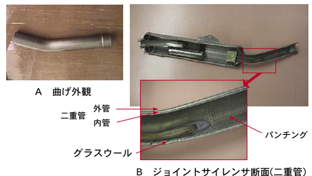
図 13 ジョイントサイレンサ曲げ外観、断面
