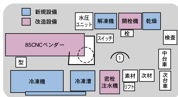
図 18 新ラインレイアウト
