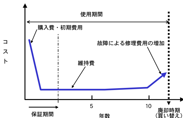
図9 コストのバスタブ曲線
