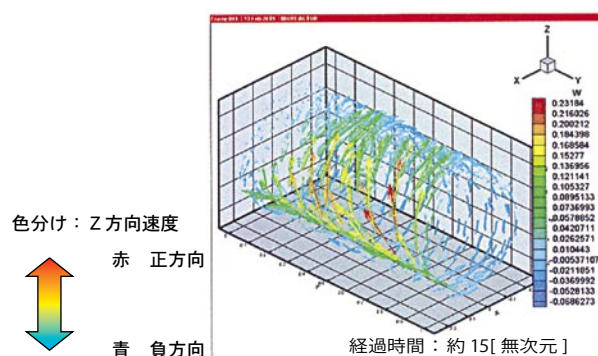
図5 バイオリアクター内の培養液の流れの様子 速度ベクトルのCFDシュミレーション結果
