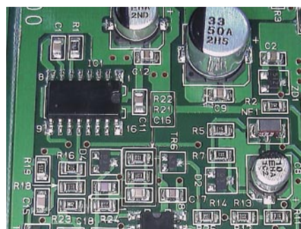
(3) 電子基板
