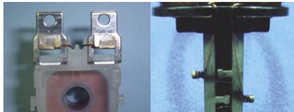
図3 電線と端子の抵抗溶接
