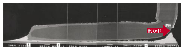
図9 ヒートサイクルによる剥がれの発生
