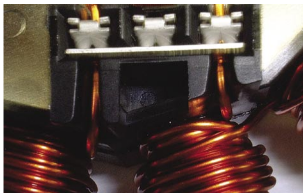
図5 かしめ端子による結線
