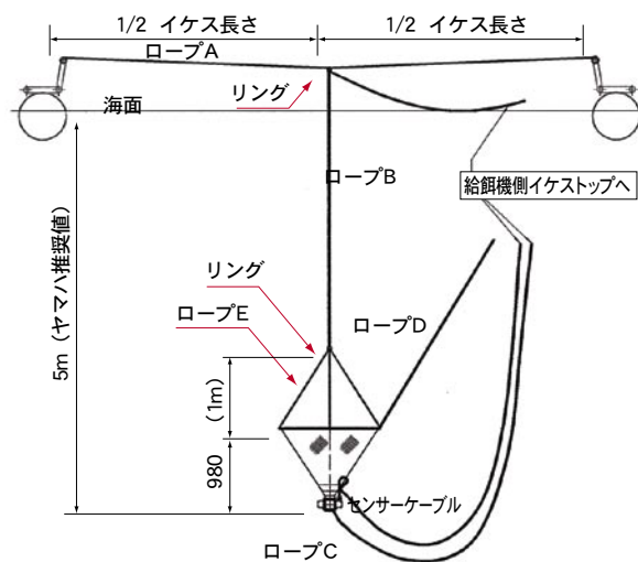
図7 残餌センサーの取り付け法
