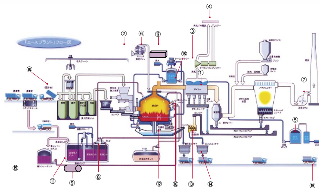
図 4 ACEP フロー図と改善項目
