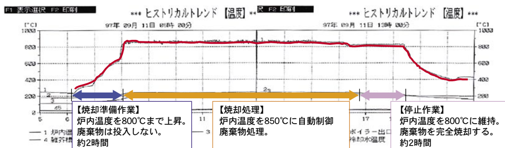
図7 ACEP 燃焼温度の変化
