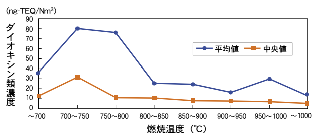
図6 燃焼温度とダイオキシン類濃度の関係
