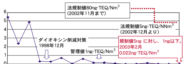
図 10 ACEP 排ガス中ダイオキシン類測定結果
