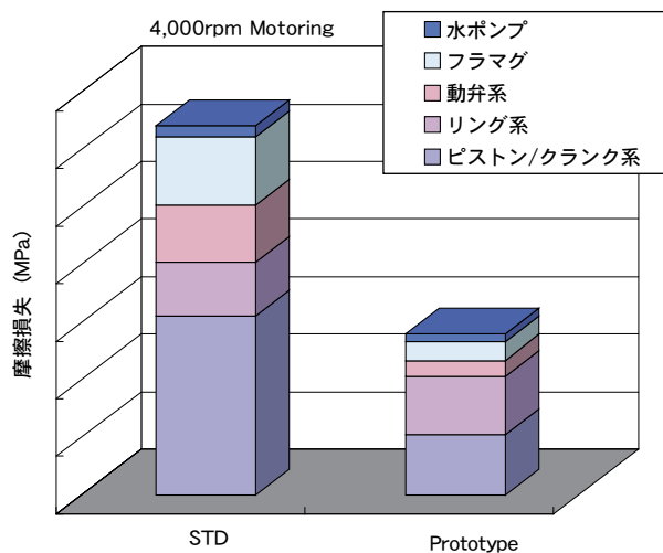
図6 摩擦損失の低減例
