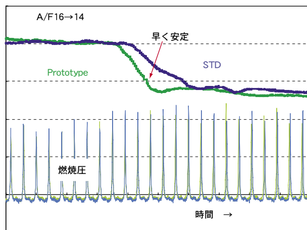
図8 改善仕様の燃料追従性比較
