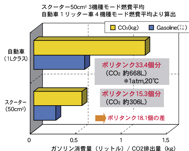
図 1 自動車とスクーターの燃費 (CO 2 排出量) 比較
