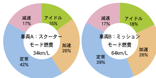
図3 運転パターン毎のモード燃費寄与
