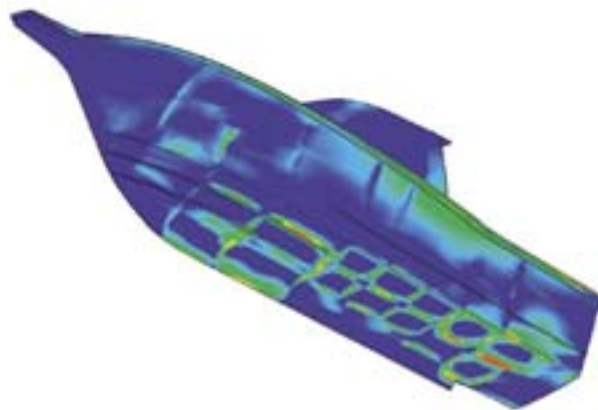
図5 FRP製艇体解析事例
