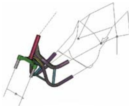
図9 車体モデル
