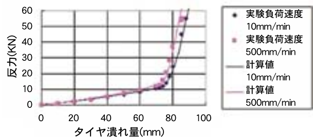
図7 静荷重
