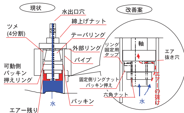
図10 耐圧栓の構造とエア残対策
