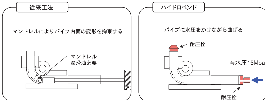
図8 工法比較
