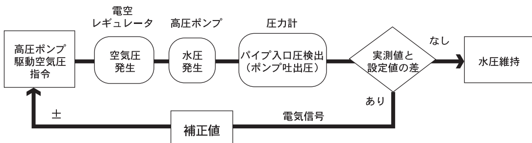
図13 高压ポンプ制御
