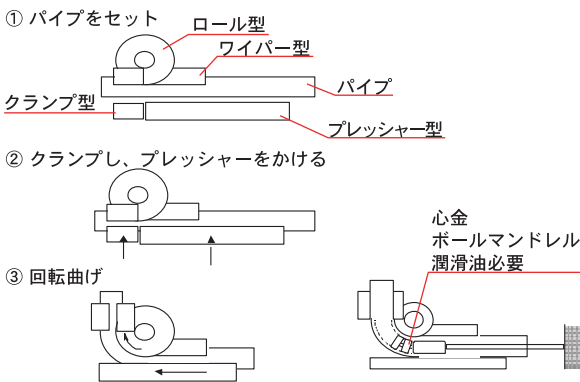
図4 回転引曲げベンダーの曲げ手順
