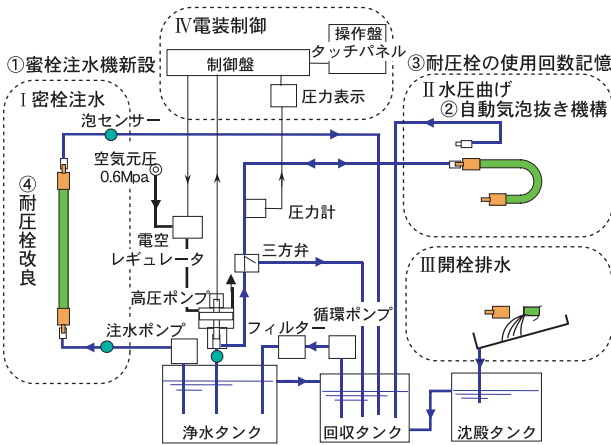
図 18 システム概要と主要な新設、改良項目
