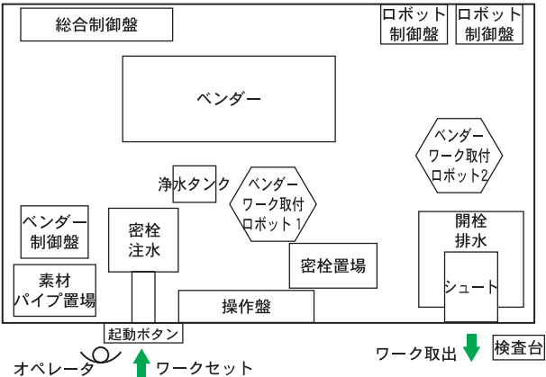
図 17 パイプ曲げ設備レイアウト
