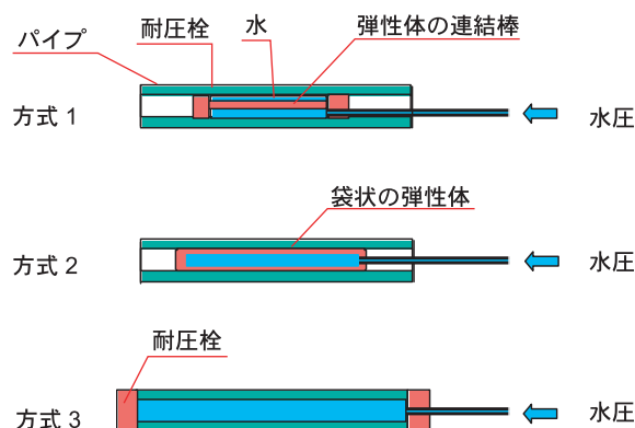
図7 水圧方式
